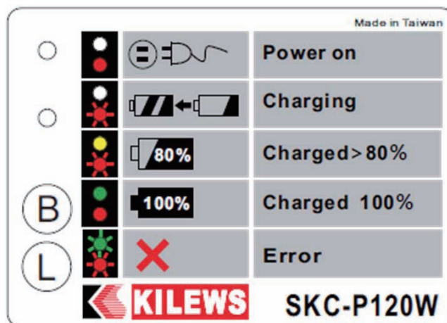
Дисплей SKC-P120W
