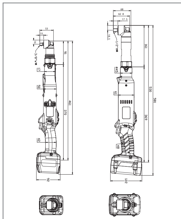
Габаритные размеры
