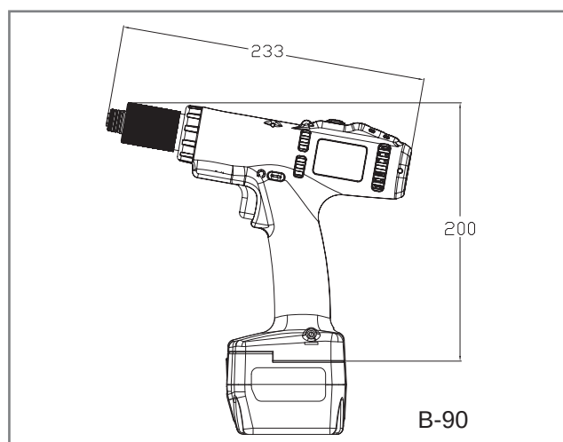
Габаритные размеры
