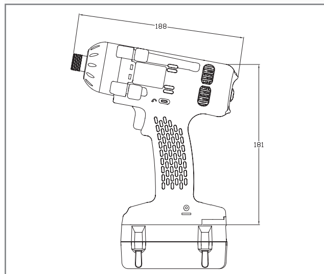
Габаритные размеры
